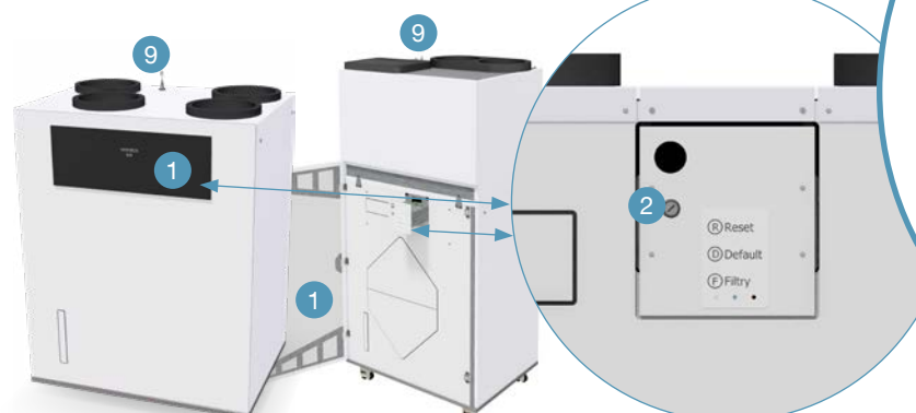
VENTBOX 800
