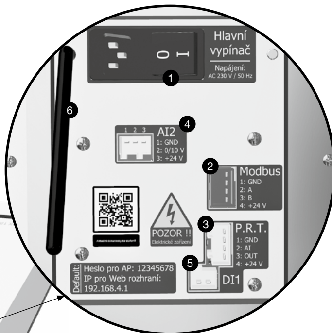
Panel řízení s připojením pro konektory
