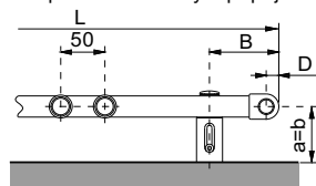
KLM, KLC, KLT bez spodního středového připojení
