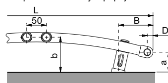
KRM, KRC, KRT bez spodního středového připojení
