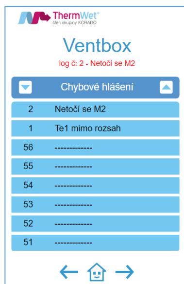
Obr. 25: Chybové hlášení
