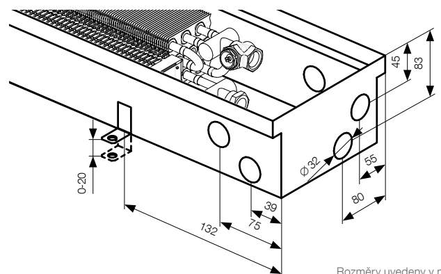
Rozměry uvedeny v mm.
