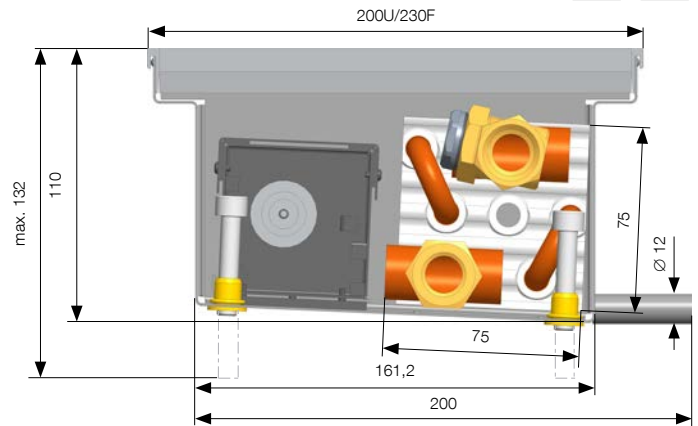
U = rámeček typu U, F = rámeček typu F. Rozměry uvedeny v mm.
