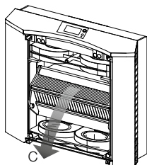
Bild 10 Wärmetauscher ausklappen
