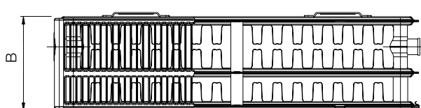
Typ 33 PLAN/LINE
