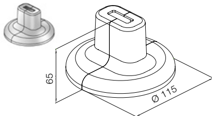
Z-U450 Grundplattenabdeckung für Innenkonsole - Universal (Z-U331)
